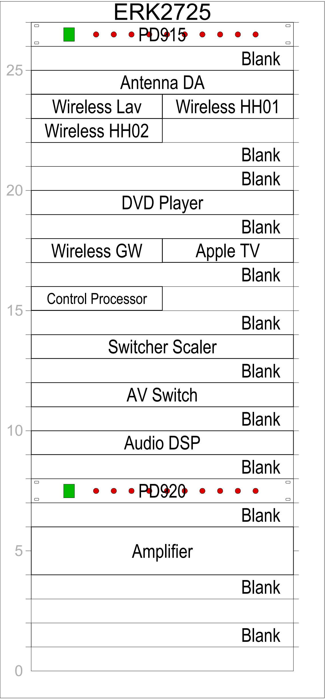
2 AV Rack Detail Scale: 3" = 1'-0"
