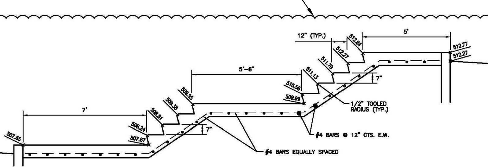
STAIR DETAIL #2 SOUTH EDGE OF STAIRS N.T.S.
