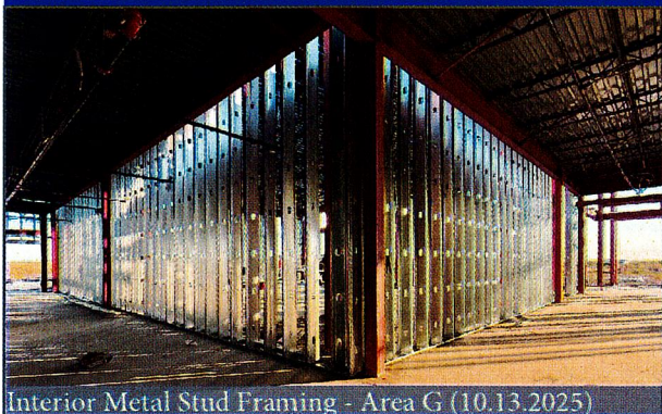
Interior Metal Stud Framing - Area G (10.13.2025)
